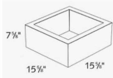
PN – 910205 16" Column
