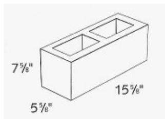
PN – 910350 6" Partition
